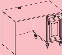
ÇALIŞMA MASASI G:106 Y:75 D:62 cm 20.21.1107.00
