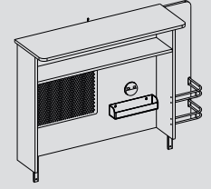
DAR ÇALIŞMA ÜNİTESİ G:109 x Y:72 x D:30 cm 20.54.1102.00
