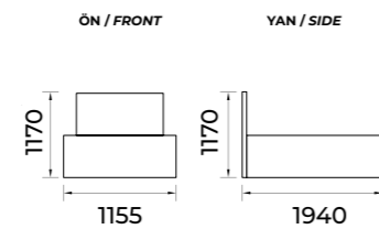
KARYOLA / BEDSTEAD
