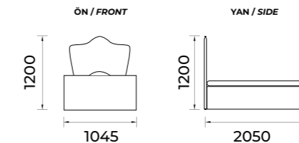
KARYOLA / BEDSTEAD
