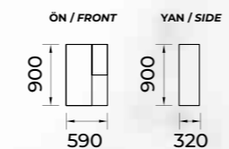
DUVAR MODÜL / WALL UNIT
