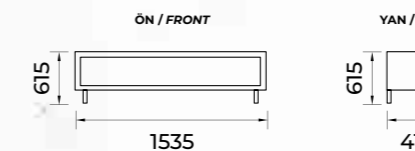
TV ÜNİTESİ / TV UNIT 2
