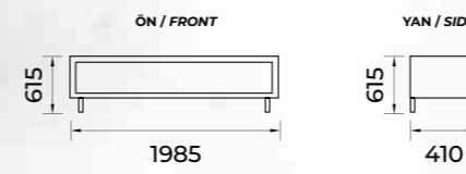
TV ÜNİTESİ / TV UNIT 1
