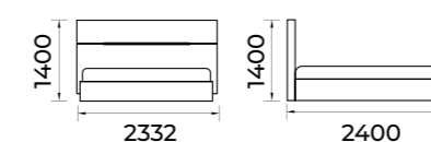
KARYOLA (PANOSUZ) / BEDSTEAD
