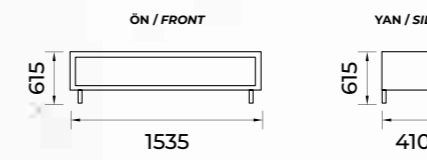
TV ÜNİTESİ / TV UNIT 2
