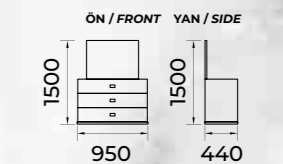
ŞIFONYER / DRESSING DESK
